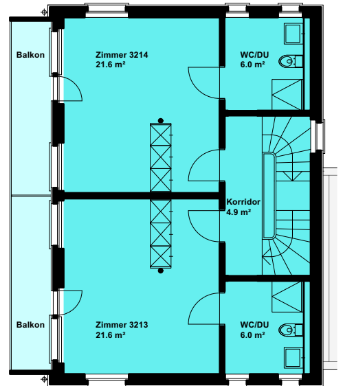
Grundriss 2.OG 1:150
