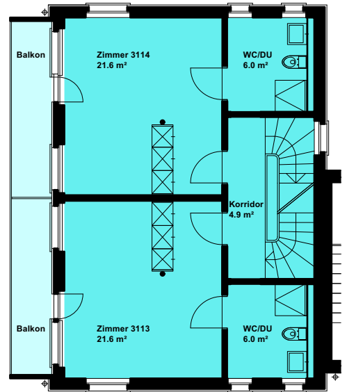
Grundriss 1.OG 1:150
